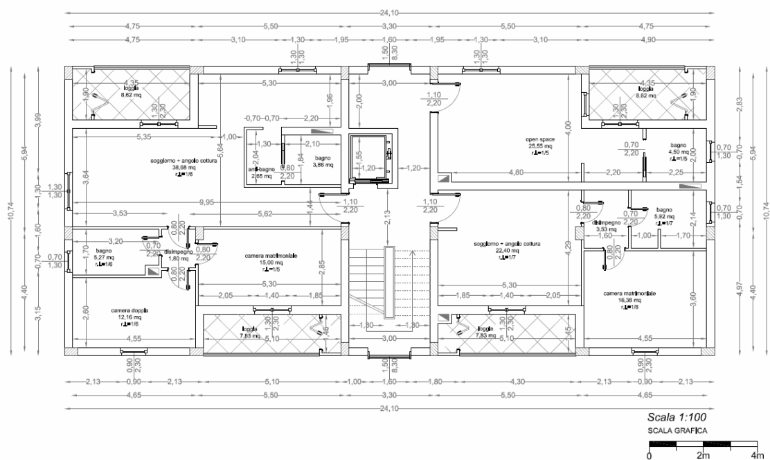
FIGURA 4. – PIANO TIPO del fabbricato residenziale.
