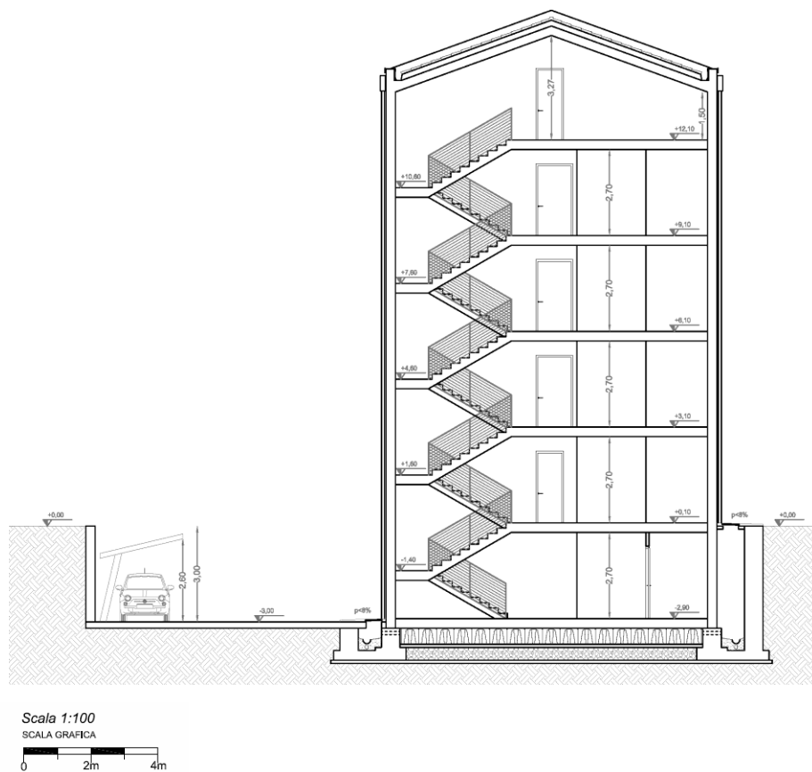
FIGURA 3. – SEZIONE LATERALE del fabbricato residenziale tipo.
